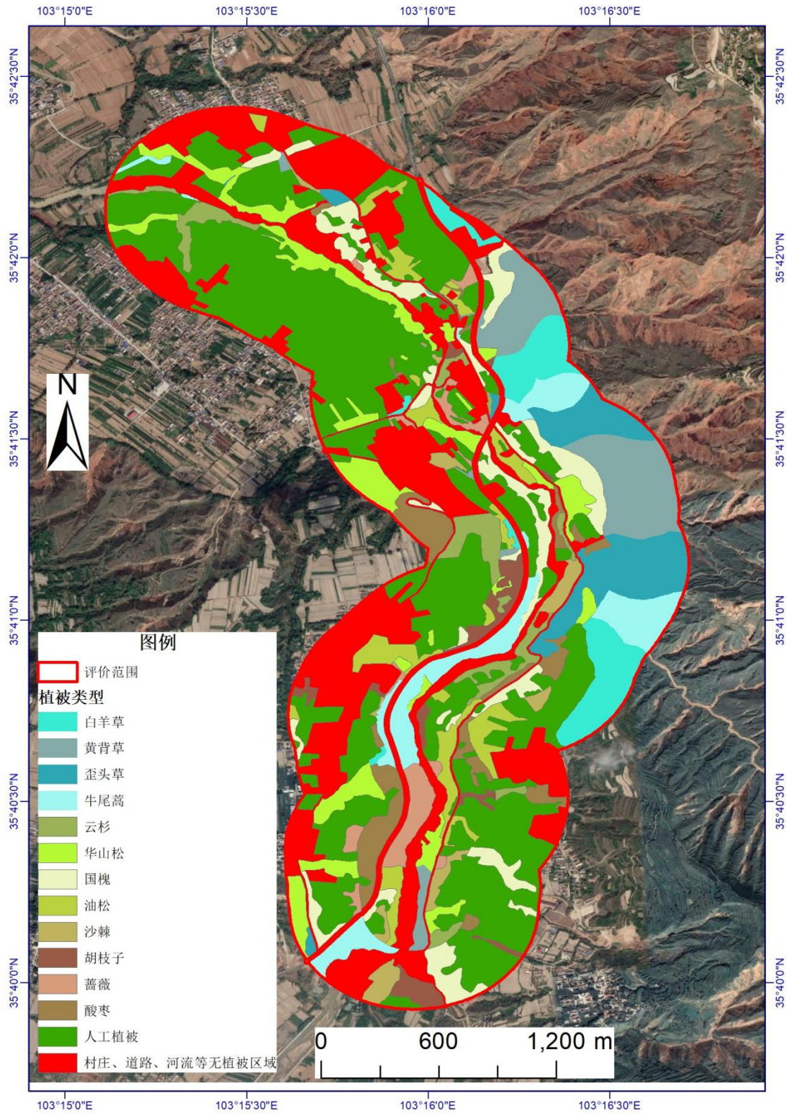
图 4-5 植被类型图
